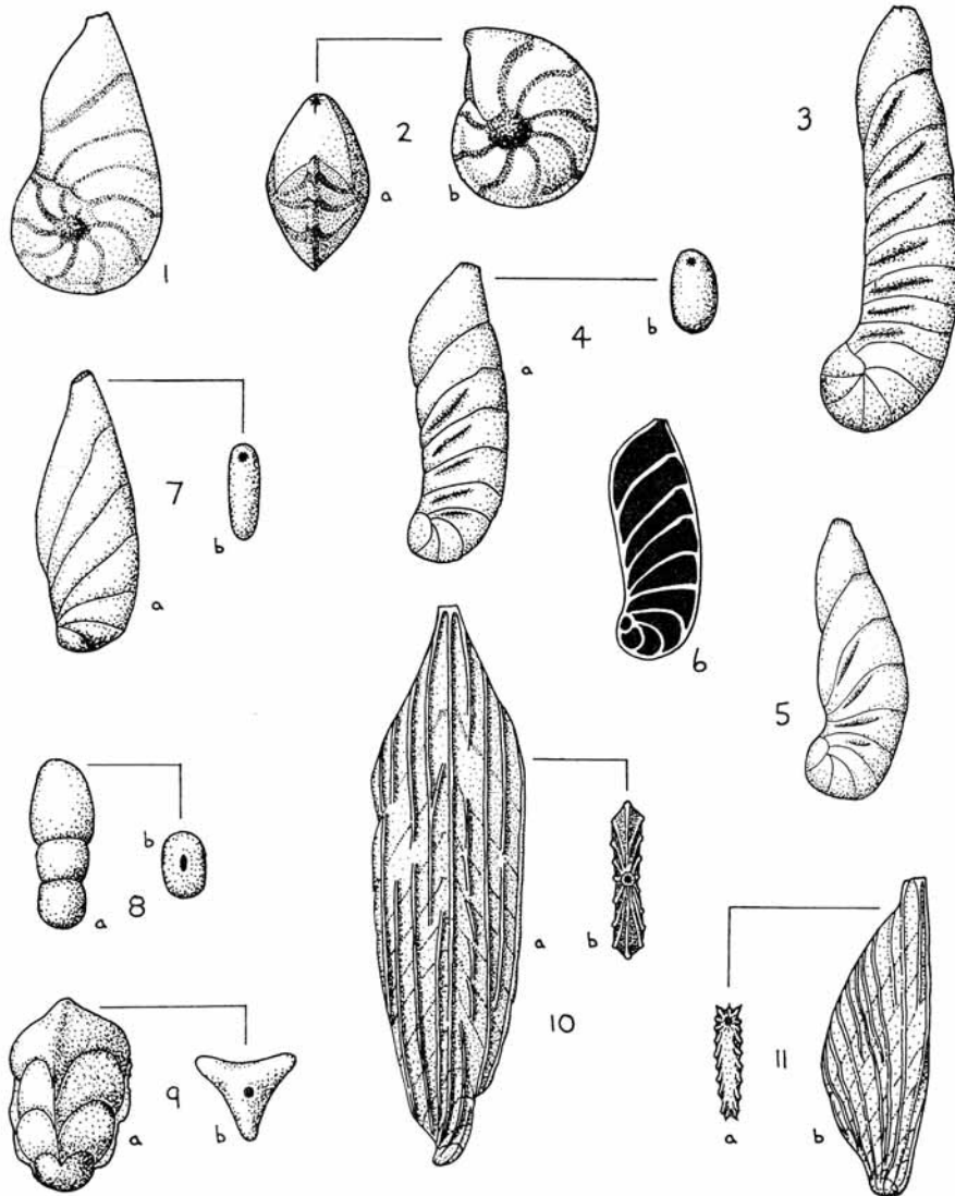
TEXT-FIG. 2. (1) Lenticulina münsteri (Roemer). Mepal. \times 40 . (2)a, b. Lenticulina münsteri (Roemer). Knapwell. \times 40 . (3) Lenticulina suprajurassica sp. nov. Holotype. Mepal. \times 40 . (4)a, b, (5) Lenticulina suprajurassica sp. nov. Paratypes. Mepal. \times 40 . (6) Lenticulina suprajurassica sp. nov. Longitudinal section. Mepal. \times 40 . (7)a, b. Planularia fraasi (Schwager). Knapwell. \times 75 . (8)a, b. Lingulina nodosaria Reuss. Knapwell. \times 75 . (9)a, b. Tristix oolithica (Terquem). Knapwell. \times 75 . (10)a, b. Falsopalmula anceps (Terquem). Knapwell. \times 40 . (11)a, b. Citharina serratocostata (Gümbel). Mepal. \times 40 .
